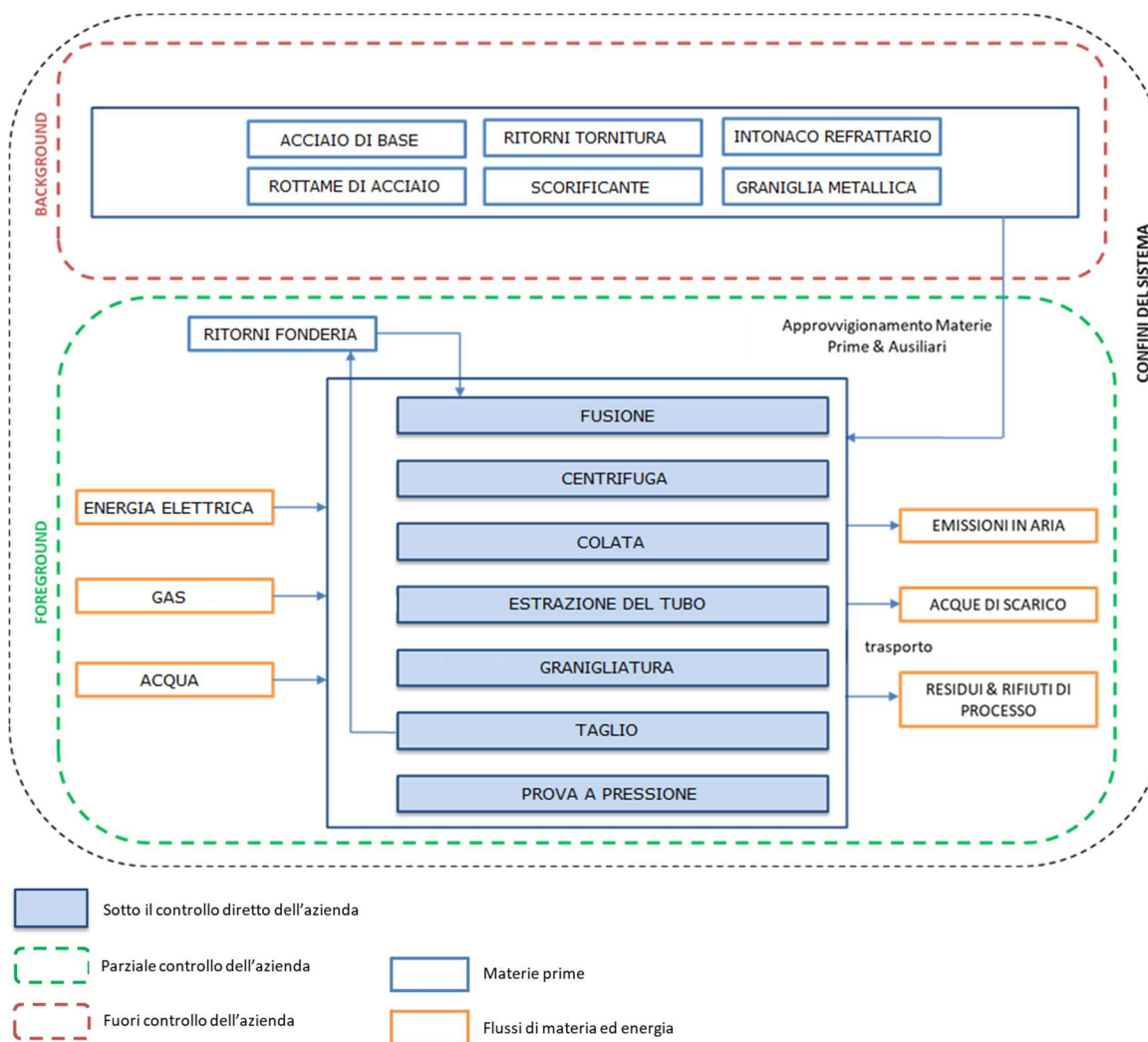
Figura 2 - Fasi del ciclo di vita e confini del sistema per i Getti di fusioni in acciaio – Stabilimento di Pontevecchio
