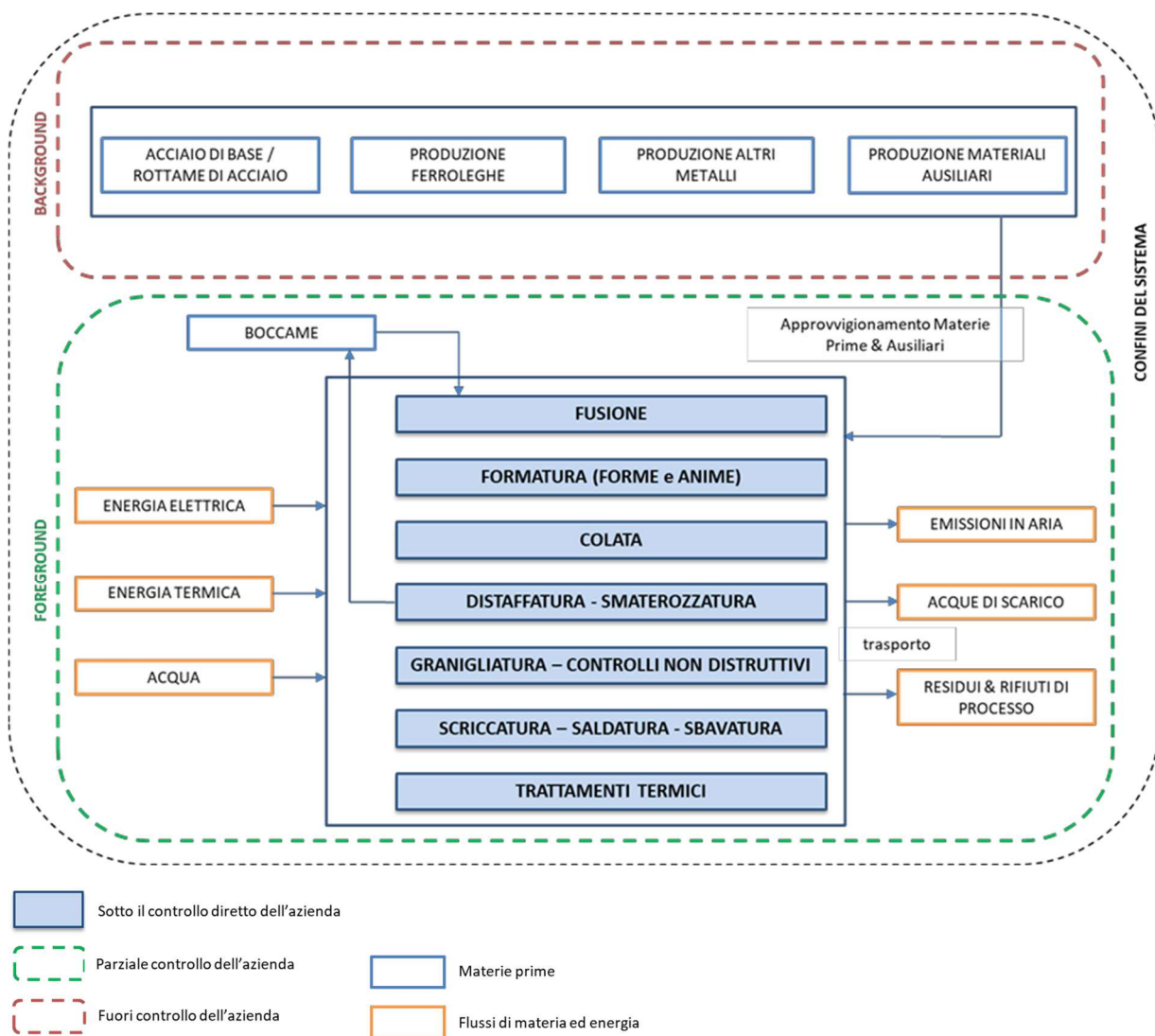
Figura 1 - Fasi del ciclo di vita e confini del sistema per i Getti di fusioni in acciaio – Stabilimento di Manerbio
